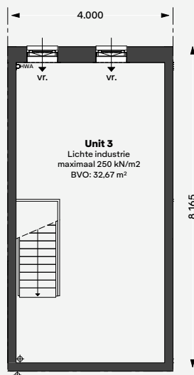
Verdieping
